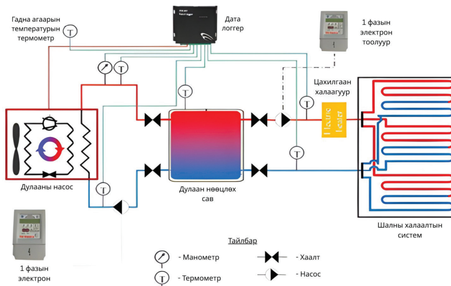
Зураг 19. Дулааны насосны ажиллагааны зарчмын схем (жишээ зураг)
