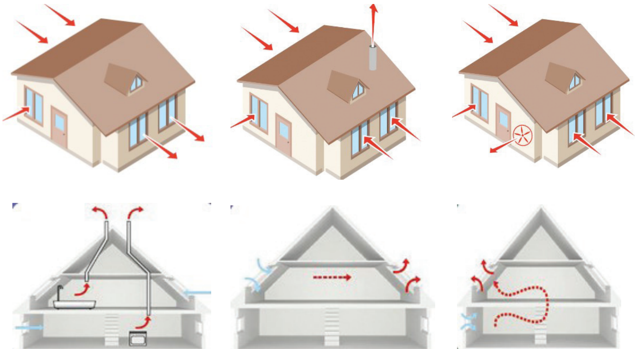
Зураг 26. Амины сууцны агаар сэлгэлтийн ерөнхий зарчим (жишээ зураг)
