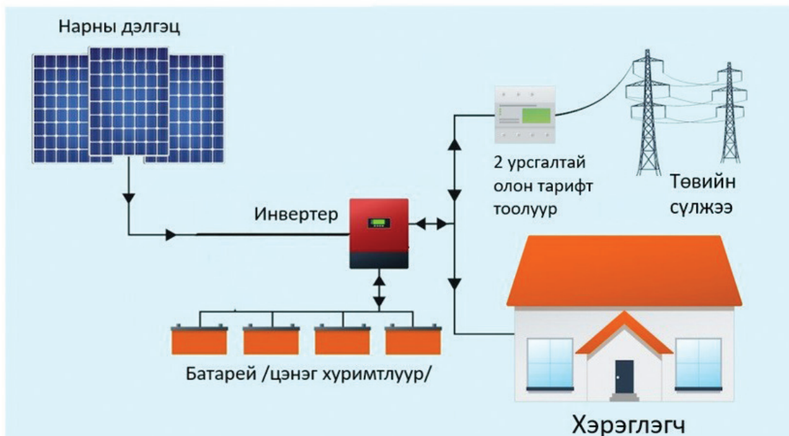
Зураг 25. Хосолмол Hybrid solar систем (жишээ зураг)
