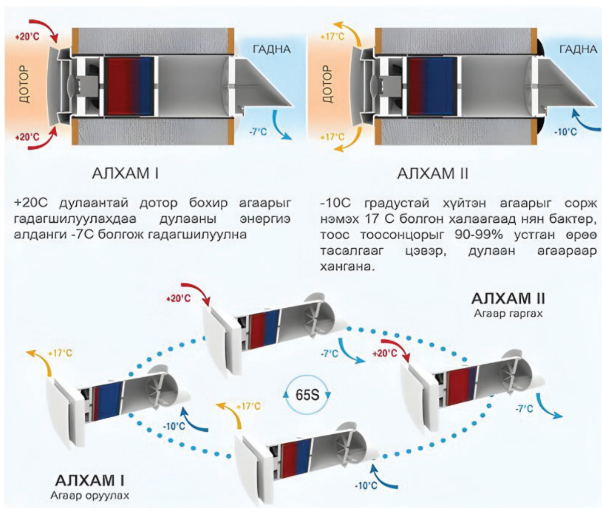
Зураг 27. Эрчим хүчний хэмнэлттэй агааржуулалтын ажиллах горим (жишээ зураг)
