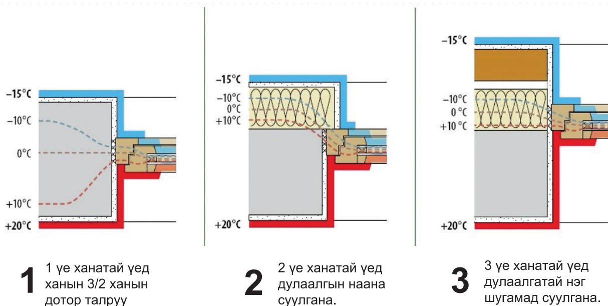
Зураг 17. Эрчим хүчний хэмнэлттэй цонх (жишээ зураг)
