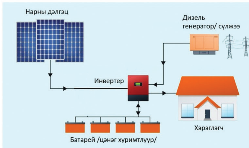
Зураг 24. Бие даасан батарейтай offgrid solar систем (жишээ зураг)
