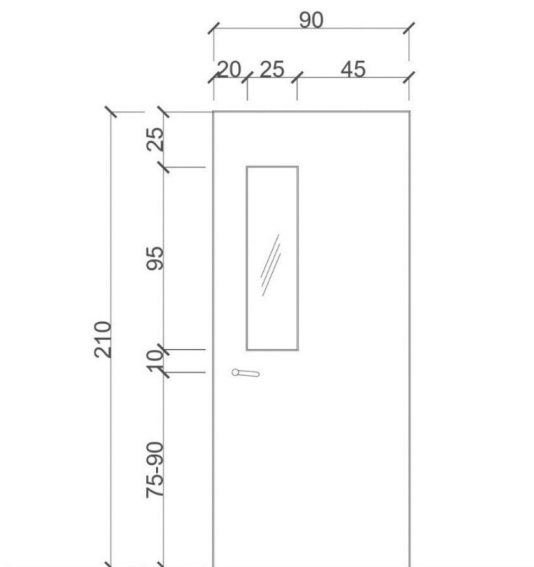
Зураг 4. Дотор хаалганы хэмжээс (жишээ зураг)
