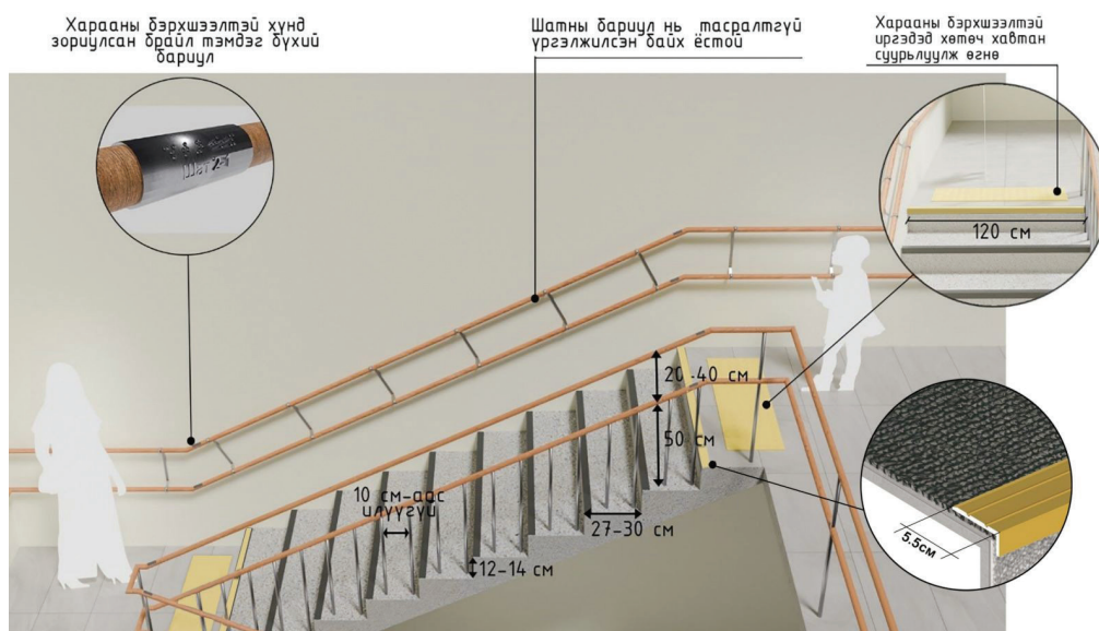
Зураг 2. Шатны стандарт (жишээ зураг)
