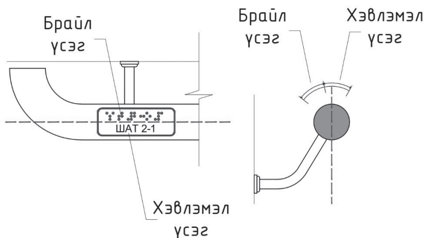
Зураг 3. Брайл тэмдэглэгээг шатны бариул дээр суурилуулах (жишээ зураг)
