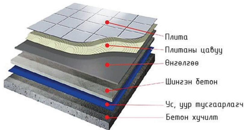
Зураг 1. Ариун цэврийн өрөөний шалны хэсэглэл (жишээ зураг)
