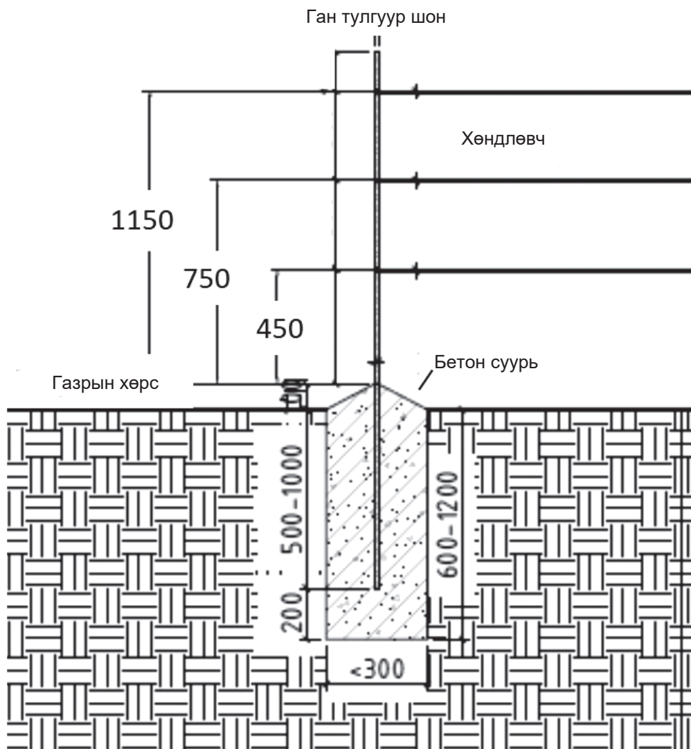
Зураг 3. Хашааны тулгуур шонгийн суурь (жишээ зураг)
