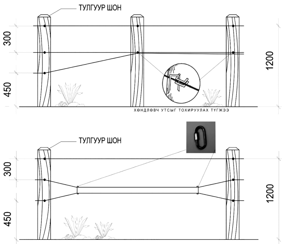
Зураг 2. Хөндлөвч утасны тохиргоо (жишээ зураг)
