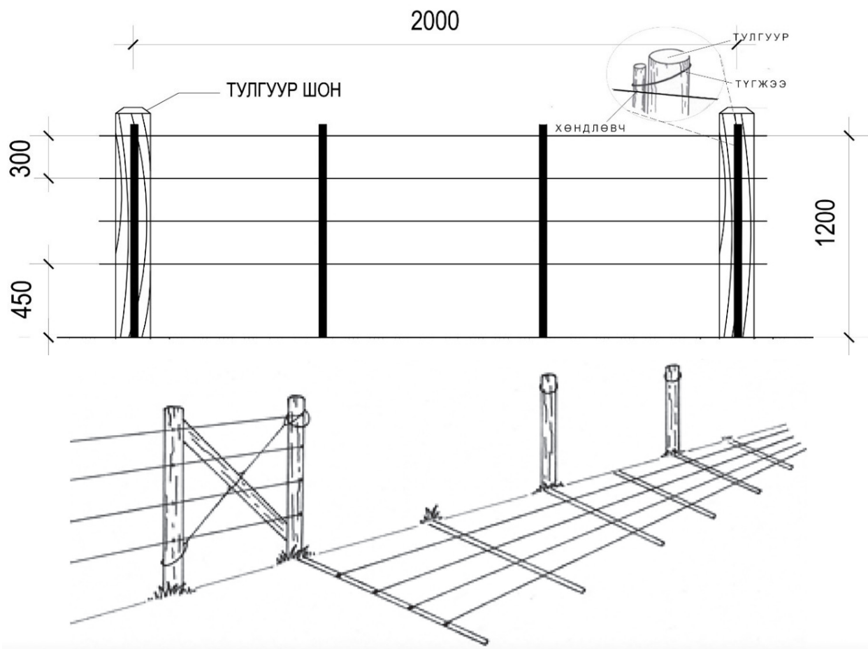
Зураг 9. Буулгадаг хашаа (жишээ зураг)
