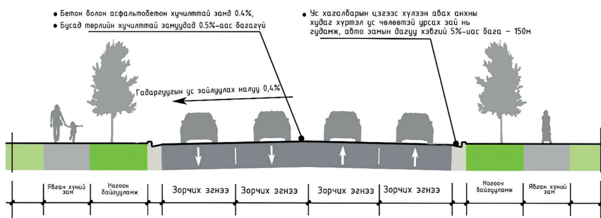
Зураг 10. Зорчих хэсгийн эгнээний налуу (жишээ зураг)
