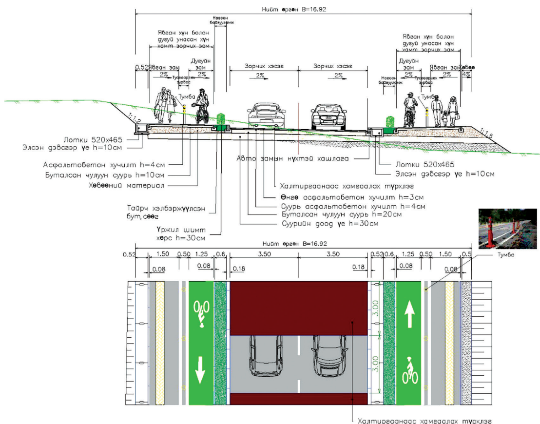
Зураг 15. Нэг хэв маягийн огтлол (жишээ зураг)
