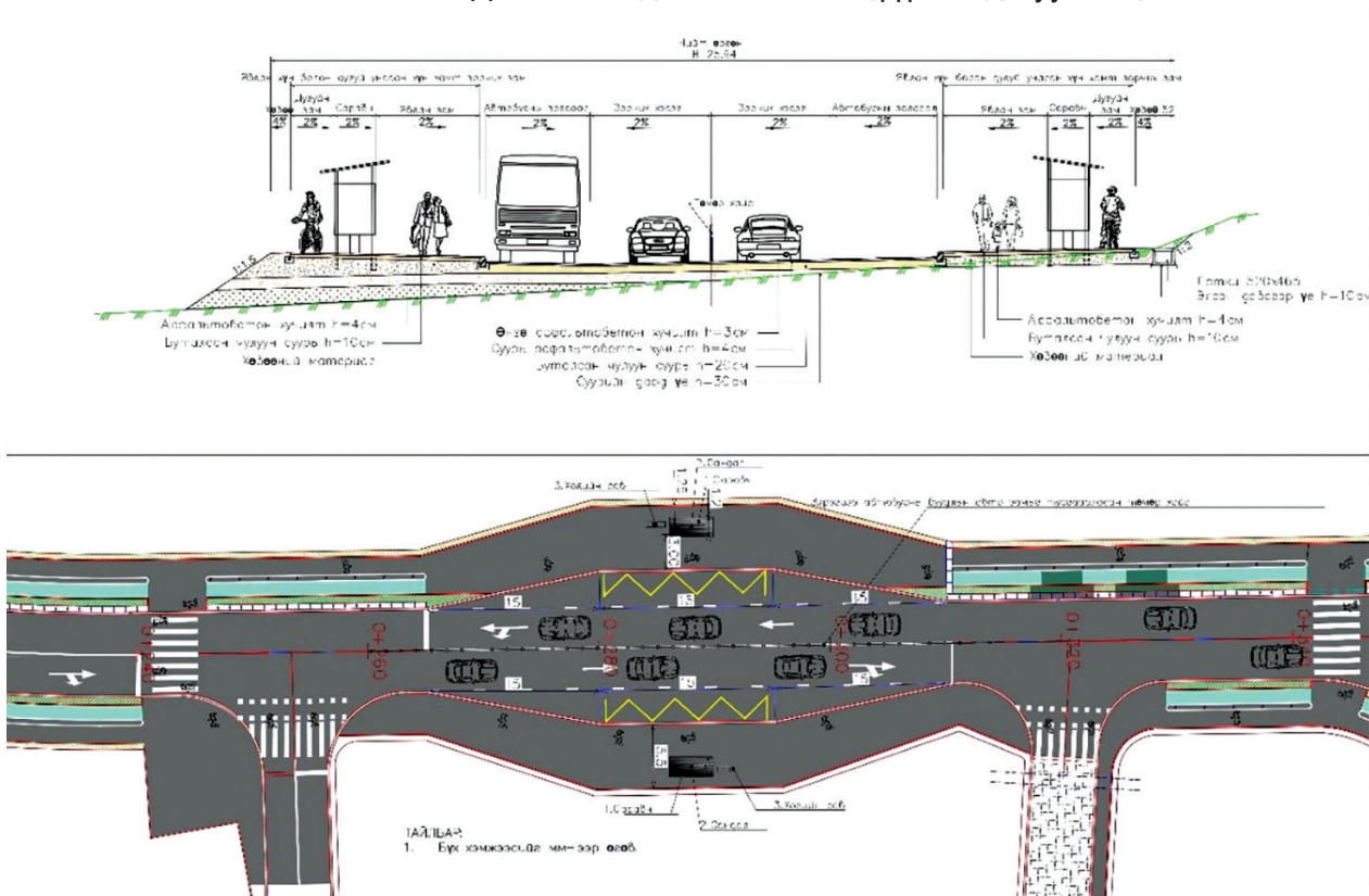
Зураг 8. Замналын зогсоолын төлөвлөлт (жишээ зураг)
