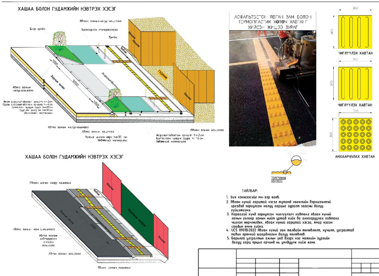
Зураг 11. Гэр хорооллын гудамж, замын орц гарц төлөвлөлт (жишээ зураг)
