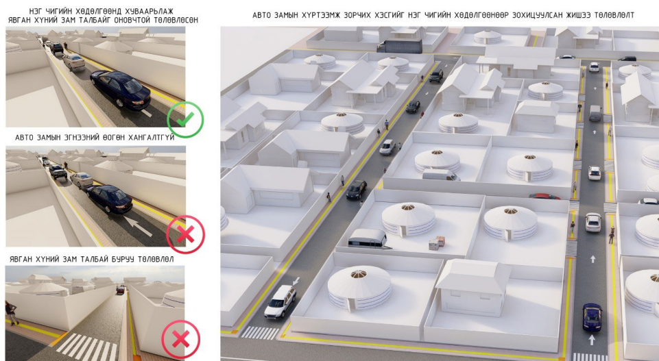
Зураг 12. Гэр хорооллын гудамж замын төлөвлөлт (жишээ зураг)
