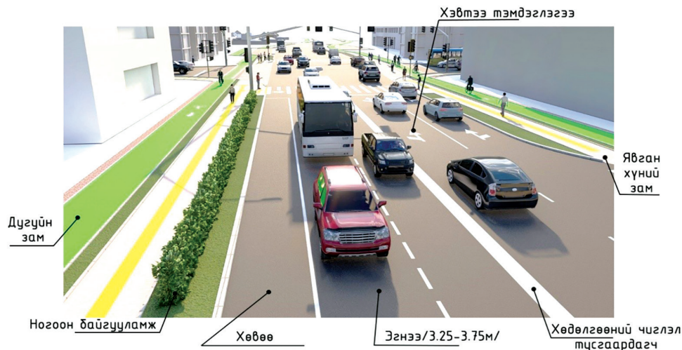
Зураг 7. Замын хөвөө (жишээ зураг)
