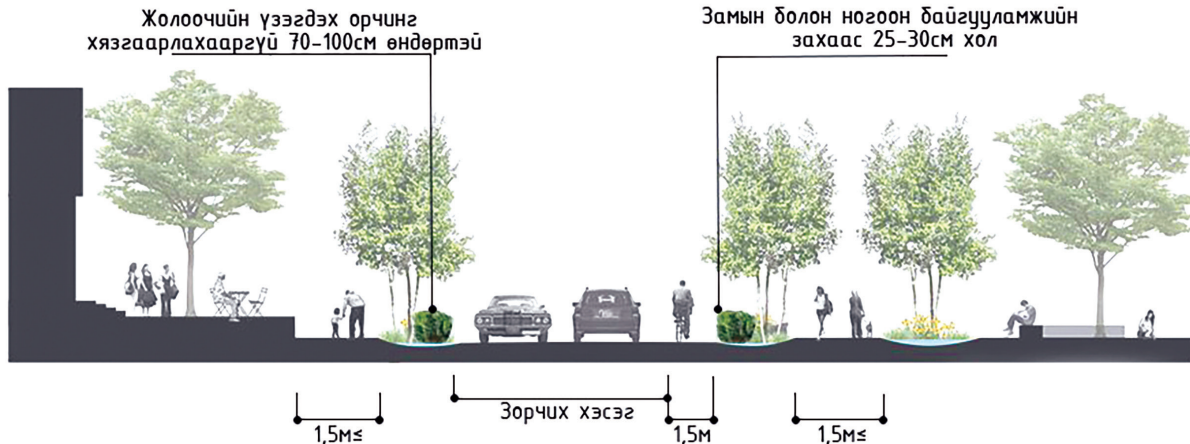
Зураг 3. Ногоон байгууламжийн тохиромжтой зай ба өндөр (жишээ зураг)
