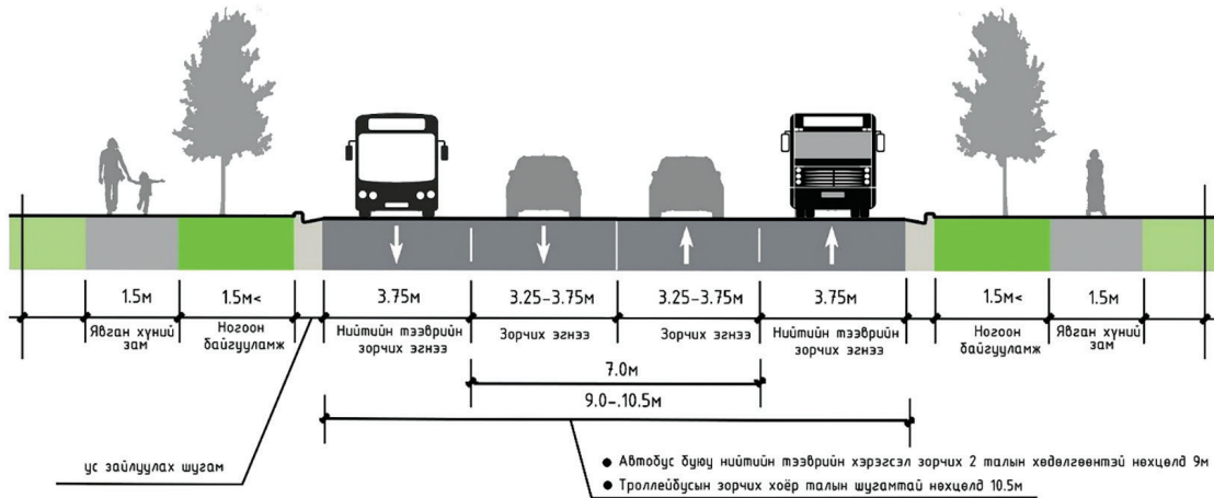
Зураг 5. Нийтийн тээврийн хэрэгслийн зорчих хэсэг эгнээний төлөвлөлт (жишээ зураг)
