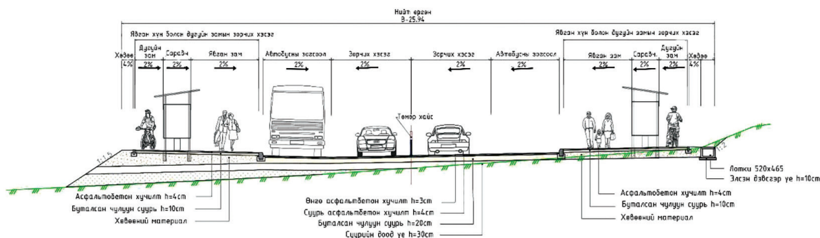
Зураг 9. Гол гудамж зам дагуу налуугийн огтлол (жишээ зураг)
