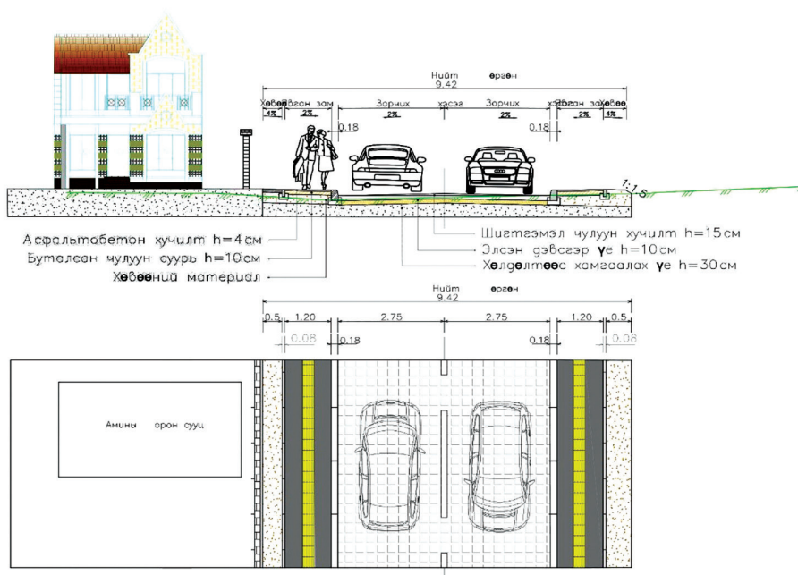
Зураг 13. Авто зам төлөвлөлт (жишээ зураг)
