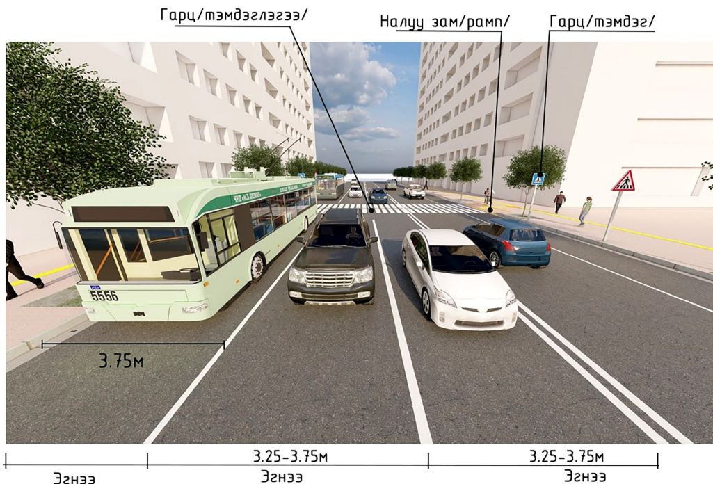
Зураг 6. Троллейбусын эгнээний өргөн (жишээ зураг)
